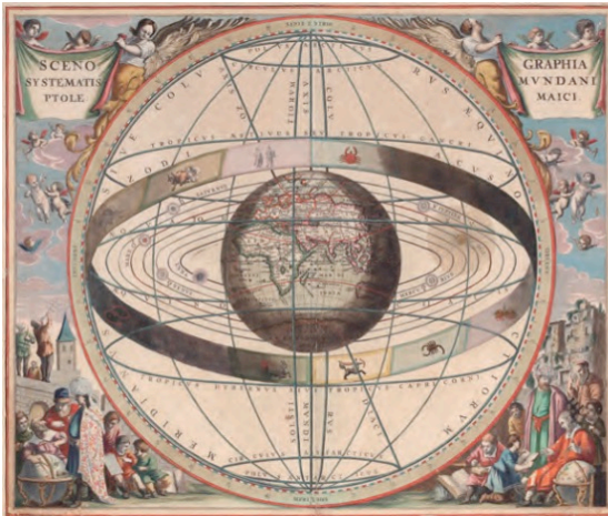
(Teoría Geocéntrica)
