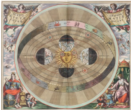
(Teoría Heliocéntrica)
